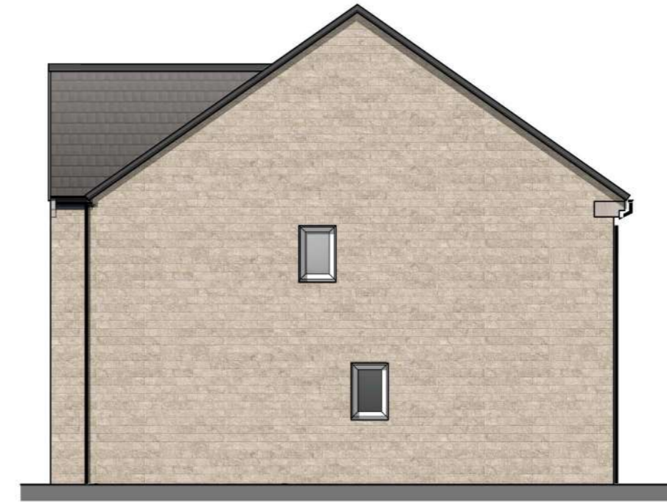
R.H.S. Elevation
