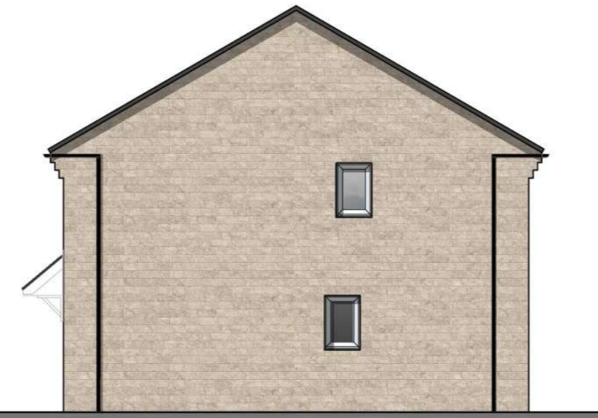
R.H.S. Elevation
